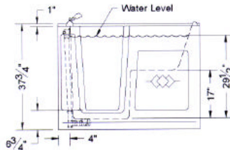
FRONT ELEVATION - SCALE: \frac{3}{8}'' = 1'-0''
