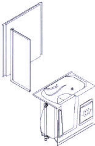
ASSEMBLY VIEW - N.T.S.
